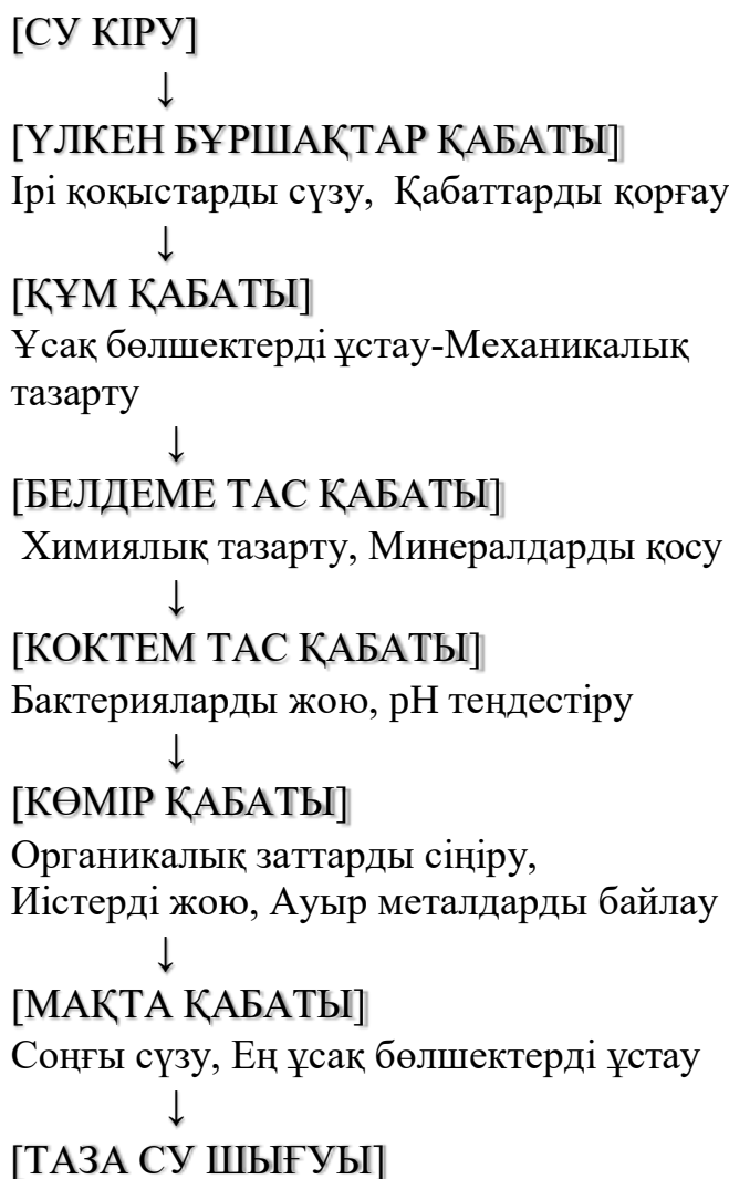
1-сурет. STEM негізіндегі су тазарту сүзгісінің жобалық моделі.
