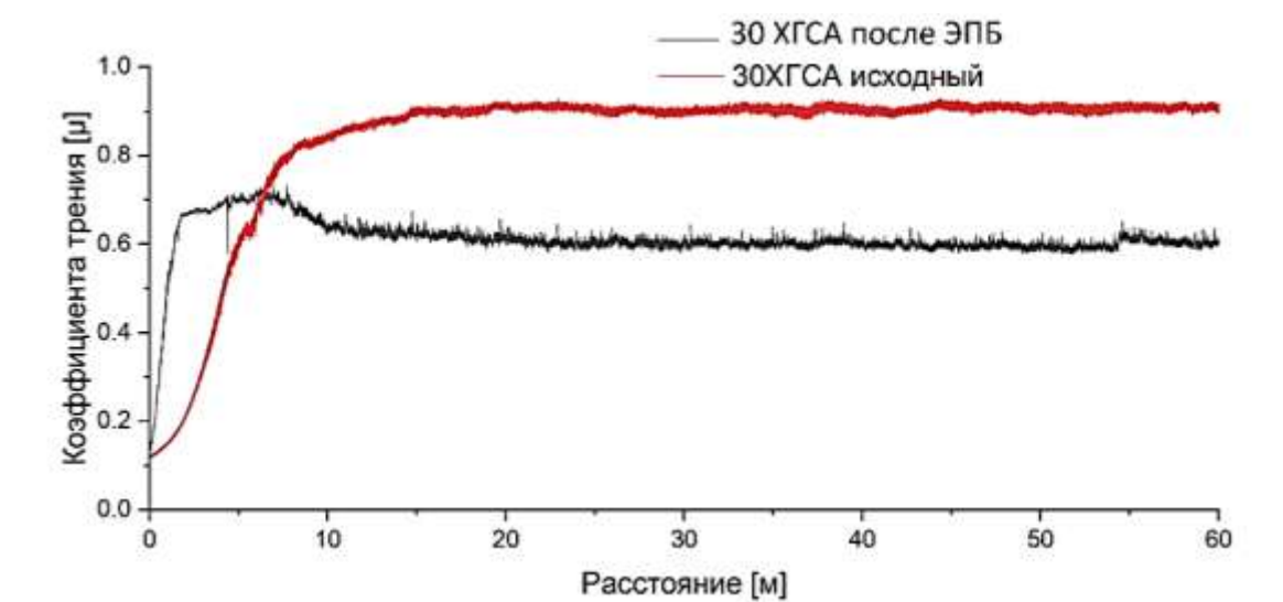
Рисунок 4. Кривые изменения коэффициента трения в процессе испытаний по схеме «шар–диск» при сухом трении для исходной стали 30ХГСА и после ЭПБ
