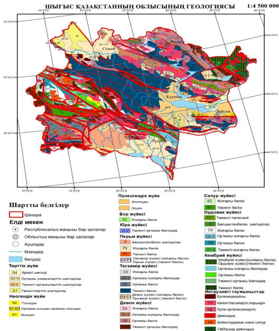
Сурет1-Шығыс Қазақстан облысының геологиясы
