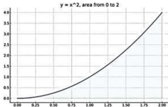
Сурет 1– f(x) = x^2 , x \in [0; 2] графигі
