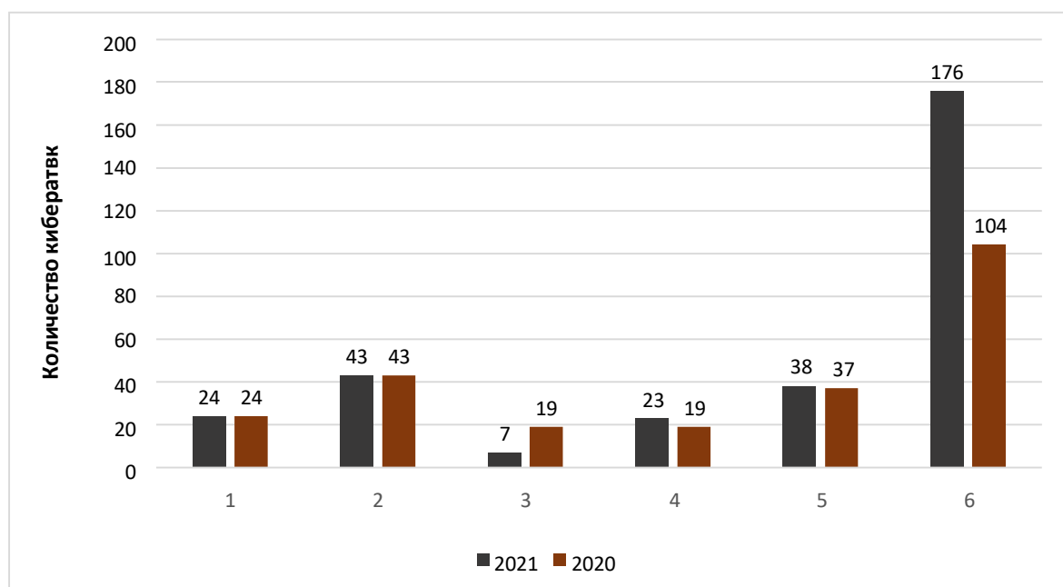
Рисунок 3 – Статистика инцидентов по видам (Условные обозначения: 1) Отсутствие доступа к информационным ресурсам; 2) Вредоносное ПО; 3) Отказ в обслуживании; 4) Несанкционированный доступ к информационным ресурсам; 5) Фишинг; 6) Другое)
