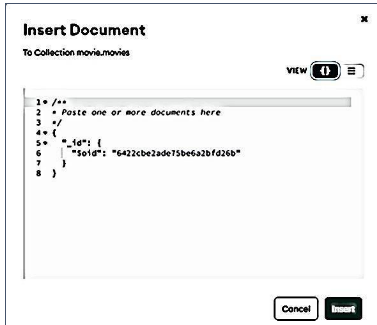
Рисунок 2- Добавление записей в БД.
