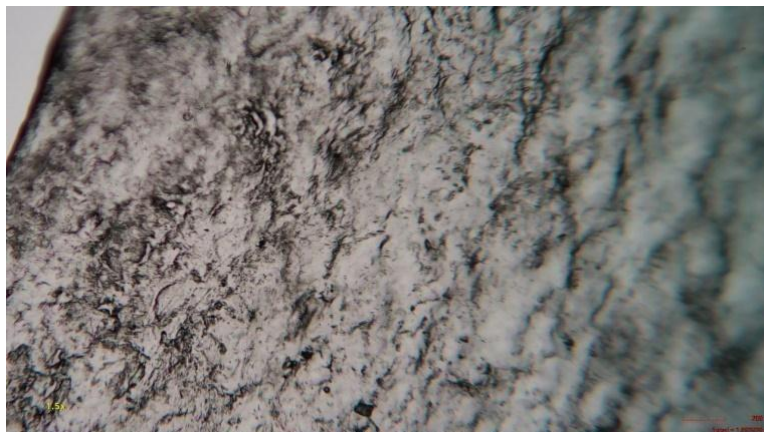
2-сурет. Тотыққан крахмал негізіндегі үлдірдің ОЭМ көрінісі
