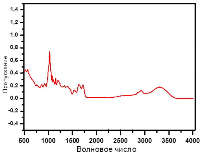
3-сурет. Тотыққан крахмал негізіндегі үлдірдің ИҚ спектрі
