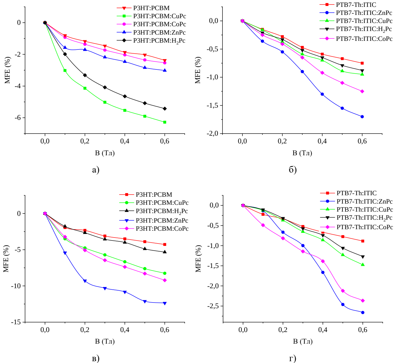
Рисунок 53 – Эффект влияния магнитного поля (MFE) на солнечные ячейки с прямой (а, б) и инвертированной (в, г) структурой
