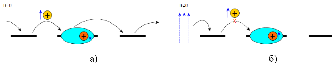
Рисунок 33 – Процесс образования биполарона
