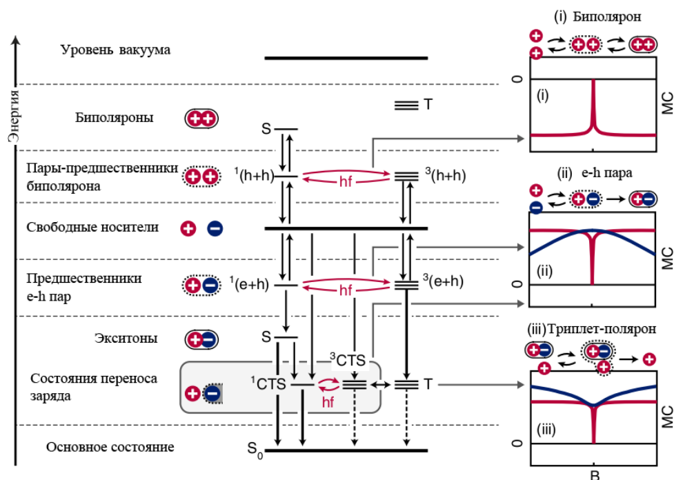
Рисунок 1– Механизмы переноса заряда в полимере
