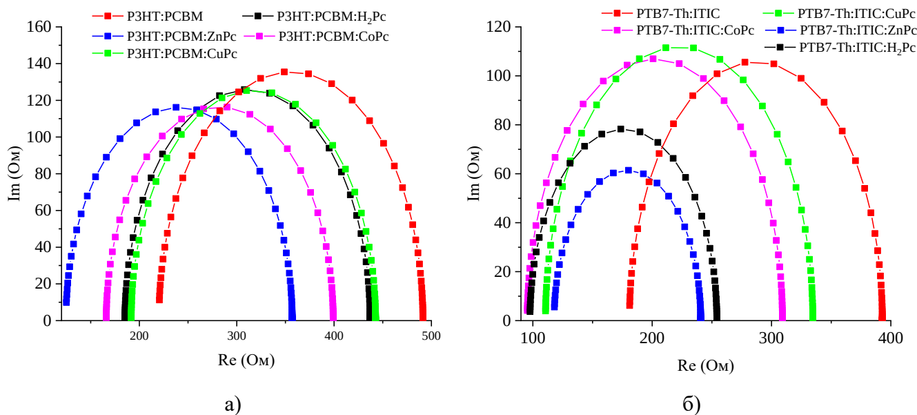
Рисунок 51 – Годографы импеданса инвертированных нанокompозитных СЯ на основе фотоактивного слоя P3HT:PCBM (а) и PTB7-TH:ITIC (б)
