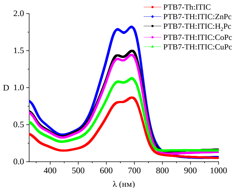
Рисунок 42 – Спектр поглощения чистого полимера PTB7-Th:ITIC и спектры поглощения нанокомпозитов PTB7-Th:ITIC, допированных нанолентами фталоцианинов
