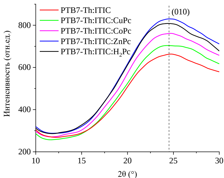
Рисунок 43 – Рентгеновские дифрактограммы нанокompозитных пленок PTB7-Th:ITIC:MPc
