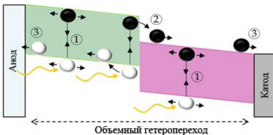
Рисунок 11 – Принцип работы солнечного элемента.
