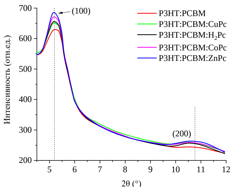
Рисунок 36 – Рентгеновские дифрактограммы нанокompозитных пленок PЗНТ:PCBM:MPc
