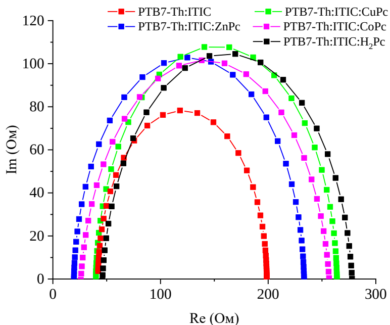
Рисунок 46 – Годографы импеданса СЯ прямой структуры на основе фотоактивного слоя PTB7-Th:ITIC и нанокомпозитов, допированных нанолентами
