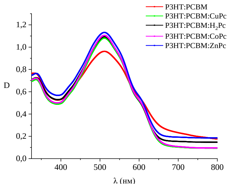
Рисунок 35 – Спектры поглощения полимера РЗНТ:РСВМ и нанокомпозитных пленок РЗНТ:РСВМ, допированных нанолентами металлофталочианинов
