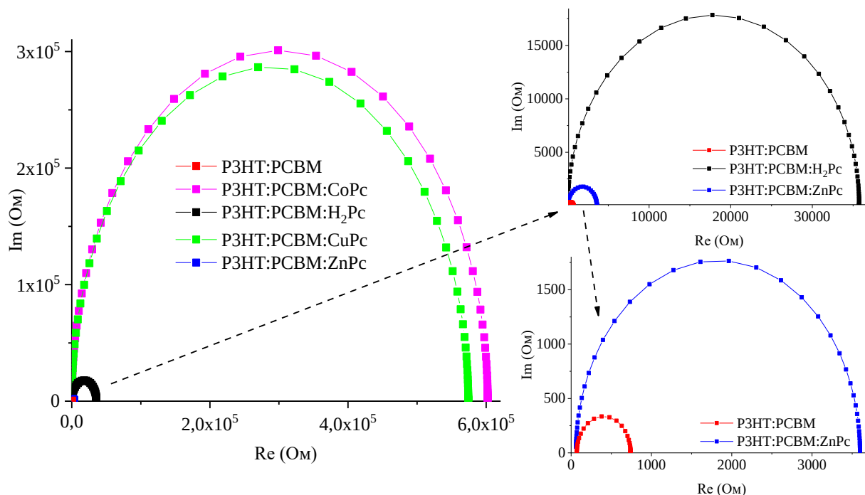
Рисунок 39 – Годограф импеданса СЯ прямой структуры на основе фотоактивного слоя РЗНТ:РСВМ и нанокомпозигов, допированных нанолентами
