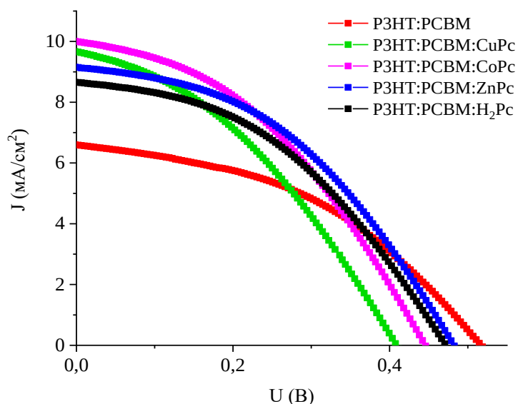
Рисунок 38 – Вольтамперные характеристики нанокомпозитных солнечных ячеек на основе РЗНТ:PCBM:MPc
