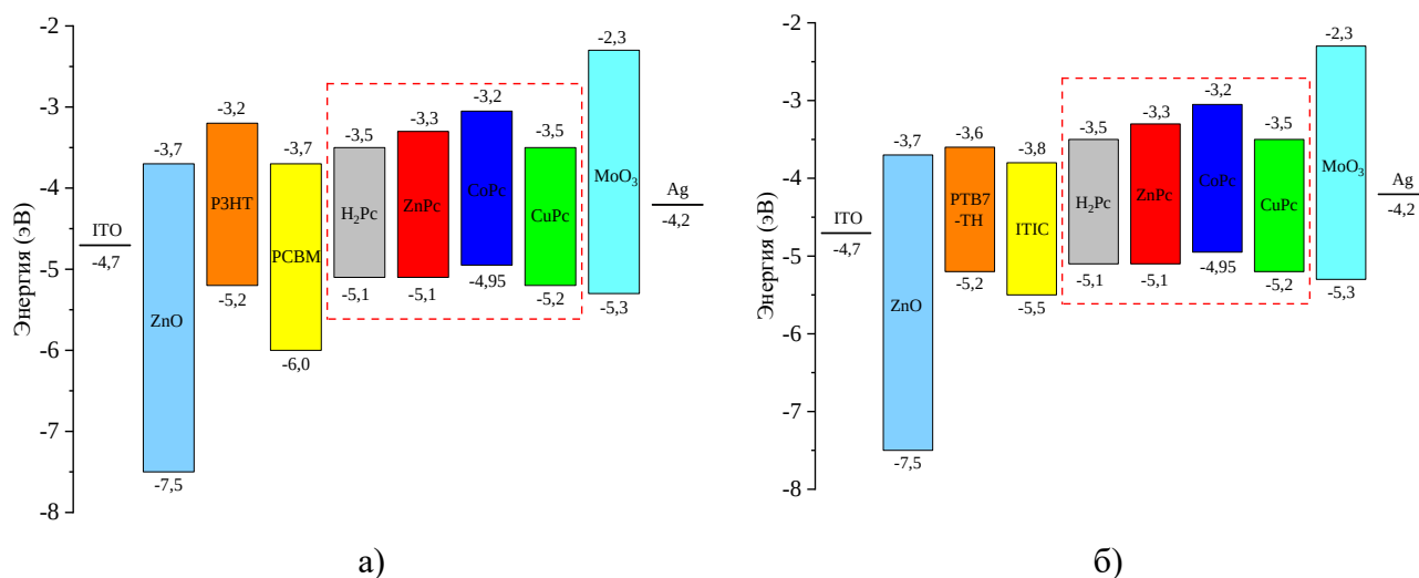
Рисунок 49 – Диаграмма энергетических уровней смеси нанокмпозитов инвертированной структуры, где МРс – CuPc, CoPc, H 2 Pc или ZnPc
