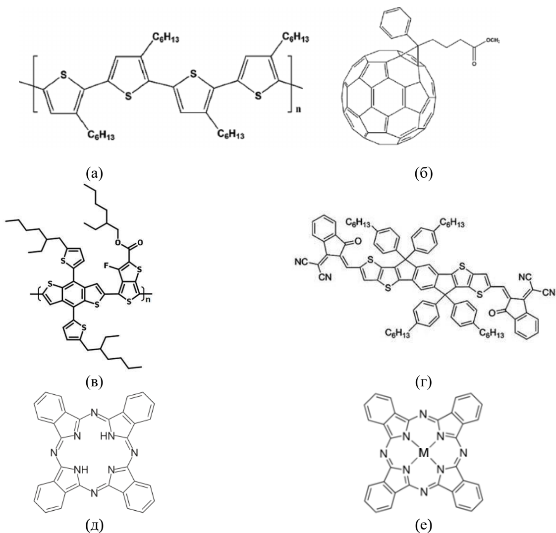
Рисунок 16 – Структурные формулы доноров РЗНТ (а) и РТВ7-Тн (в); акцепторов РСВМ (б) и ИТIC (г); фталоцианина (д) и металлокомплексов фталоцианина (е) (где М – Cu, Co, H 2 , Zn)
