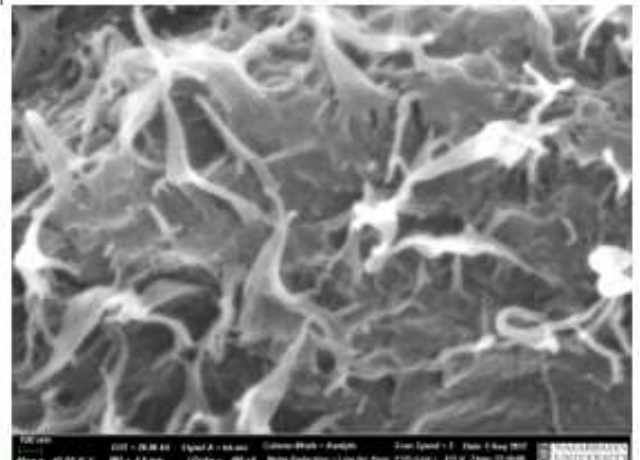
Сурет 3.15 – 30масс.% минералды диабаз толтырғышы бар АЖМПЭ микроқұрылымы
