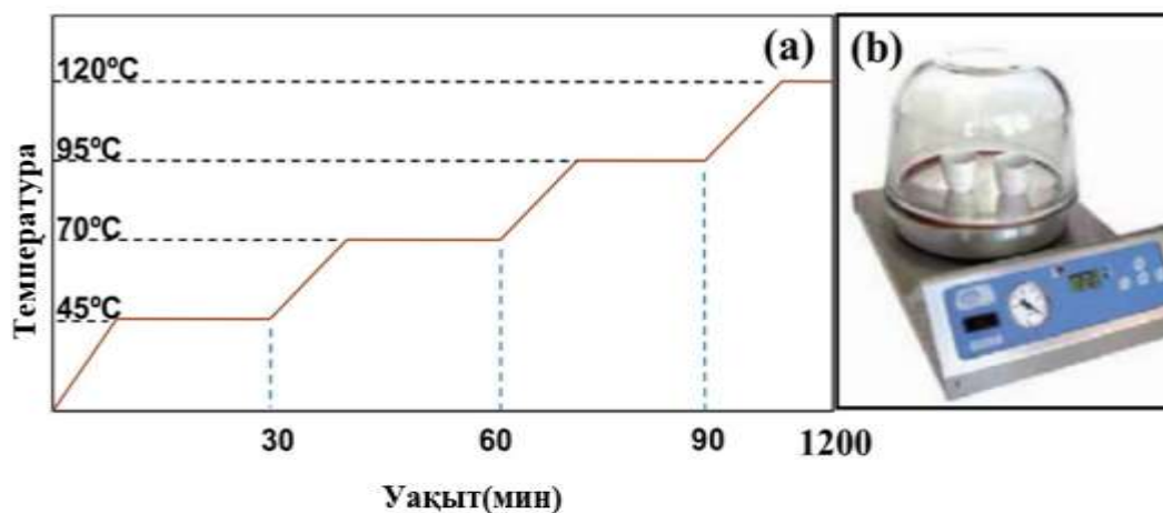
Сурет 1.12 – а) АЖМПЭ нанокөмпозициялық қаптамаларын шоғырландыру үшін пайдаланылатын кезеңнен кейінгі жылудан кейінгі өңдеу схемасы, (b) кейінгі өңдеу процесі үшін пайдаланылатын қыздыру тақтасы [79]
