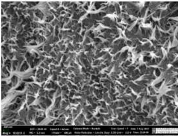
Сурет 3.15 – 30масс.% минералды диабаз толтырғышы бар АЖМПЭ микроқұрылымы
