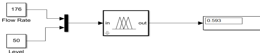
2 сурет – Мұнай деңгейін басқару жүйесін анық емес реттеудің ішкі жүйесі
