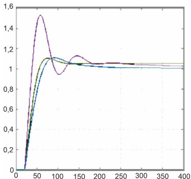
3 сурет – Өтпелі графиктер (сары график – П реттеу, күлгін график – ПИ реттеу, көк график – анық емес реттеу)
