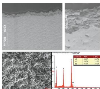
РЭМ изображения Ті/ГА покрытий
