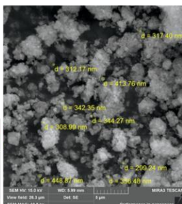
РЭМ изображения ГА порошков
