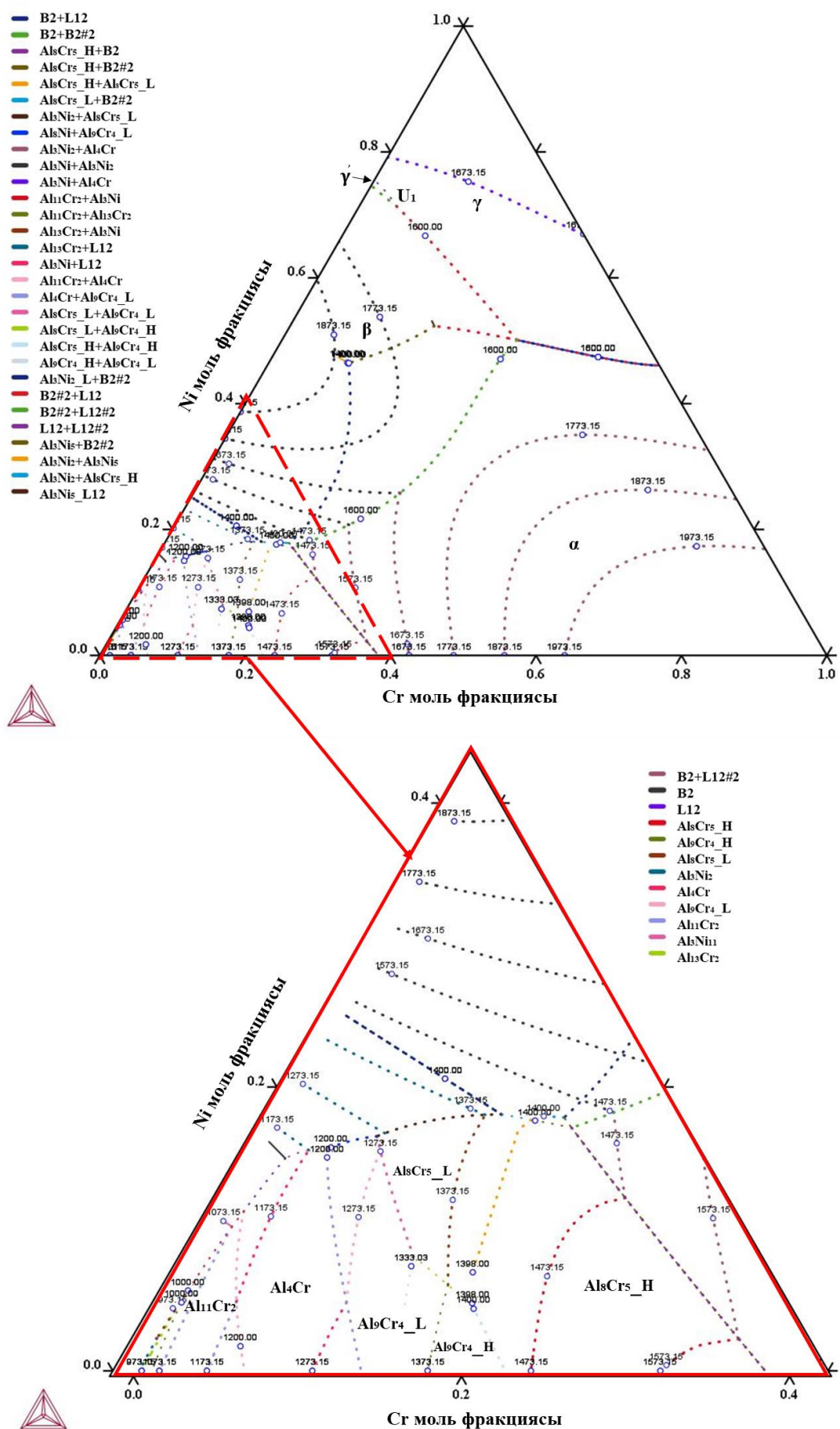
Сурет 1.4 – Ni-Cr-Al жүйесі үшін есептелген ликвидус проекциясы
