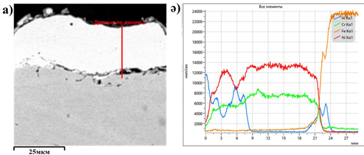
а) жабынның құрылымы; б) элементтік талдау нәтижесі
