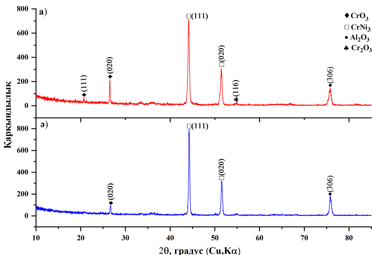
Сурет 4.25 – Өндірістік ортада жоғары температуралық сынаудан кейінгі градиентті (а) және біртекті (ә) NiCr-Al(20%) жабындарының рентген фазалық талдау нәтижелері.
