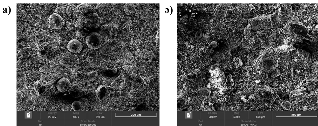
Сурет 4.24 – NiCr-Al(20%) градиентті жабындарының өндірістік ортада жоғары температураға ұшырағанға дейін (а) және кейінгі (ә) беткі морфологиясы
