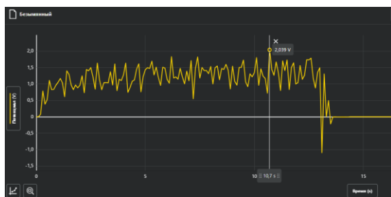
Сурет 31 - Vernier Graphical Analysis бағдарламасында алынған деректер
