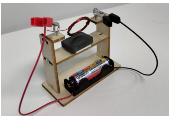
Сурет 32 - Электр тізбегінің жұмысын тәжірибе арқылы түсіндіруге арналған құрал
