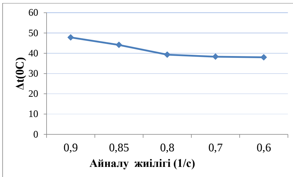
Сурет 35- Стирлинг қозғалтқышымен жасалған тәжірибе нәтижелерінің графигі
