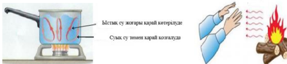
Сурет 19 – Термодинамикадағы энергия: Жылу алмасу тақырыбын оқыту
