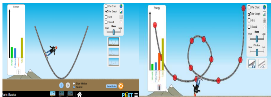
Сурет 24 - Энергияның түрленуі: кинетикалық, потенциалдық және жылулық энергия
