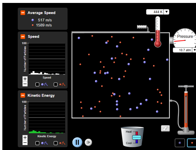
Сурет 26 - Газ молекулаларының энергиясы
