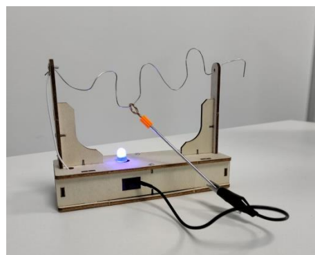
Сурет 32 - Электр тізбегінің жұмысын тәжірибе арқылы түсіндіруге арналған құрал
