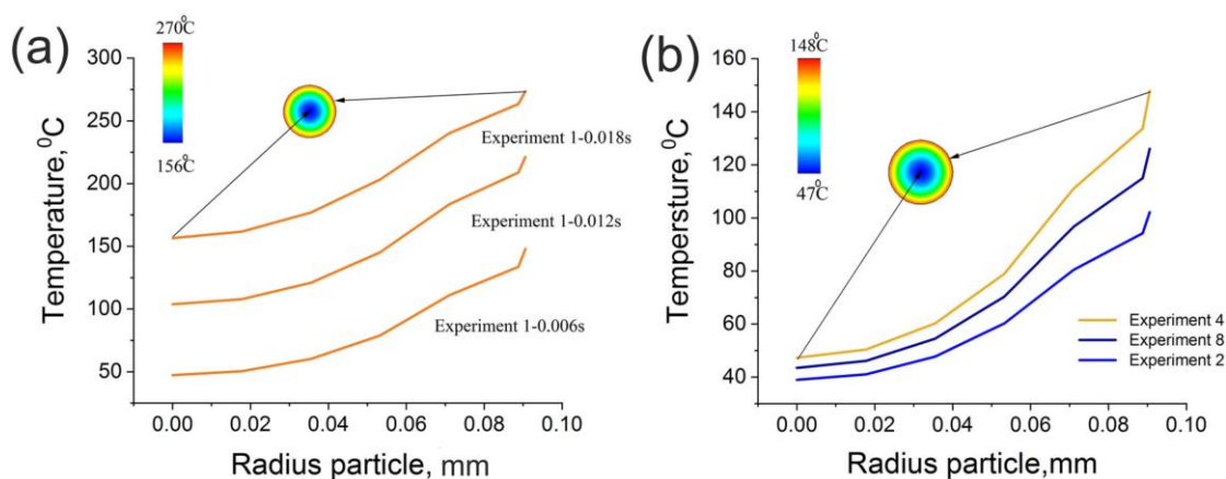
Сурет 37 – (а) Уақыт факторының УЖМПЭ бөлшектерін тұрақты температурада қыздыруға әсері. (b) 0,006 с тұрақты қыздыру уақытында бөлшектердің қызуына температура факторының әсері.
