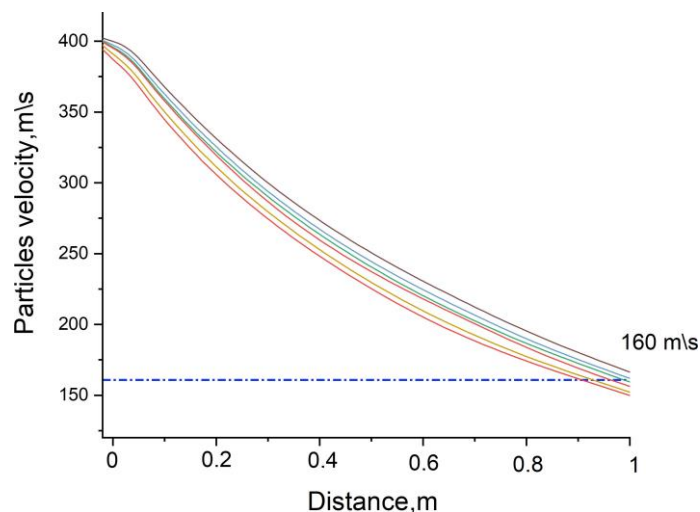
Сурет 33 – 1 бар қысымда орталық жалын осі бойымен УЖМПЭ бөлшектерінің жылдамдығының өзгеруі.
