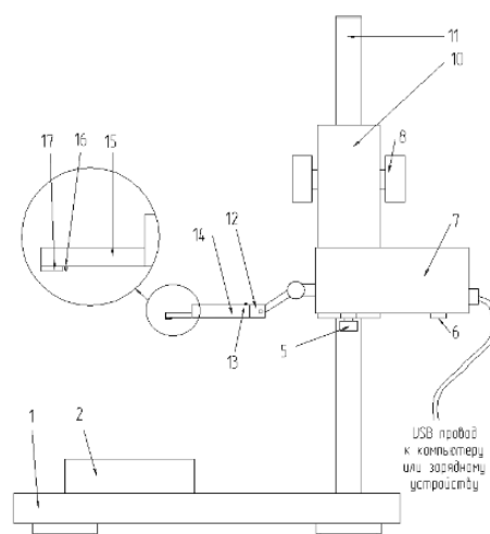
Сурет 45 – Профилометр 130 моделі
