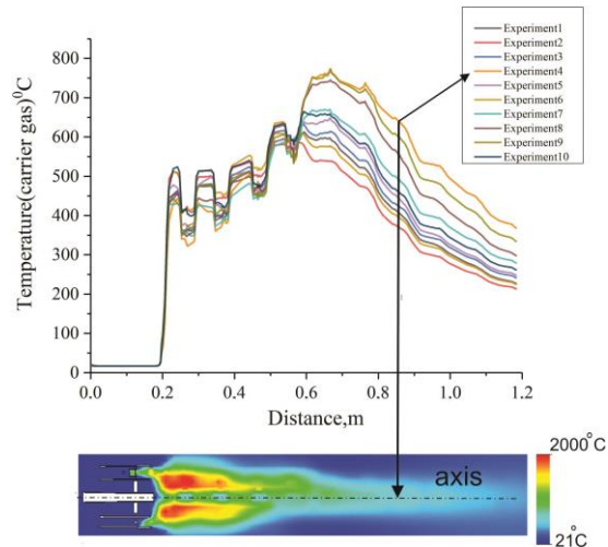
Сурет 31 – Айнымалы технологиялық параметрлердің орталық жалын осі бойындағы жалын температурасына әсері
