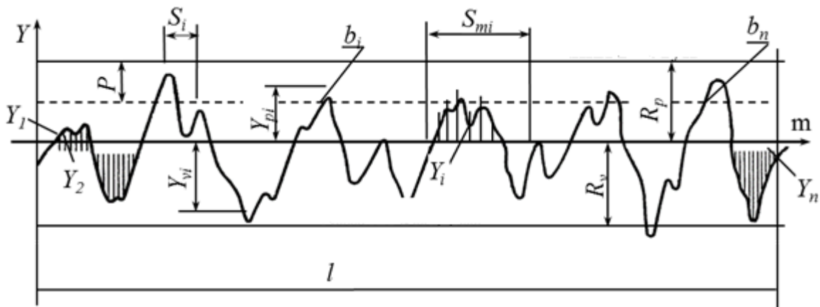
б) зерттелетін бөлшектің бойлық қимасының профилограммасы және бетінің кедір-бұдырлығының негізгі параметрлері
