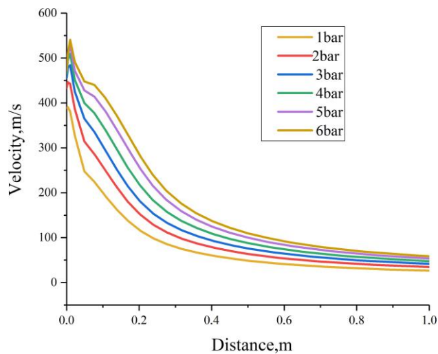
Сурет 32 – 1-6 бар қысымда орталық жалын осі бойымен тасымалдаушы газ ағынының өзгеруі.
