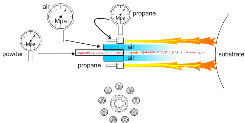
Сурет 30 – Полимерлі термопластикалық материалдарды бүркуге арналған эксперименттік қондырғының схемасы
