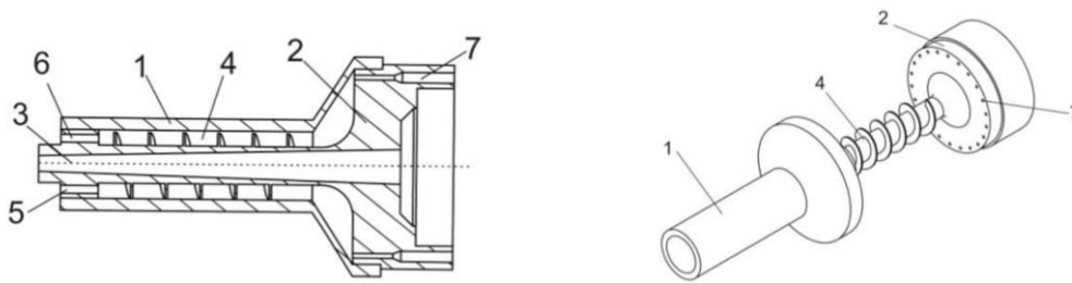
Сурет 27 – Оттықтың диаграммасы Сурет 28 – бөлшектелген көрініс
