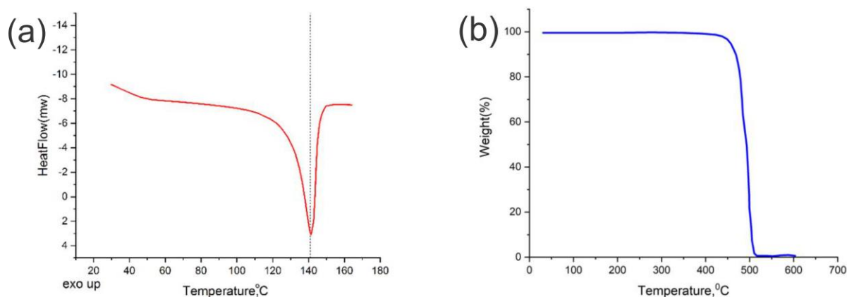
Сурет 36 – (a) УЖМПЭ ұнтағының дифференциалды сканерлеу калориметриясы. (b) УЖМПЭ термогравиметриялық талдау
