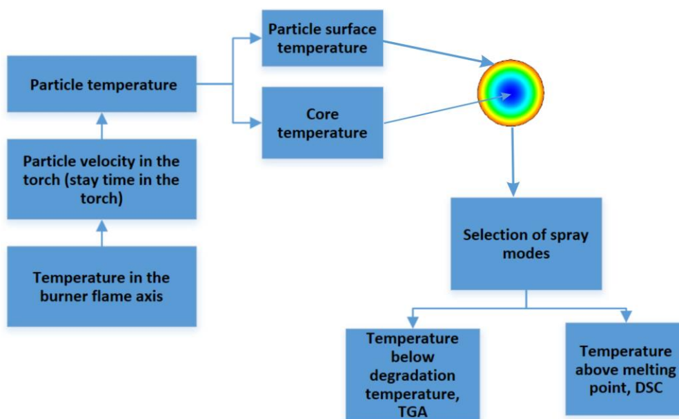
Сурет 34 – Бұрку режимін таңдау схемасы
